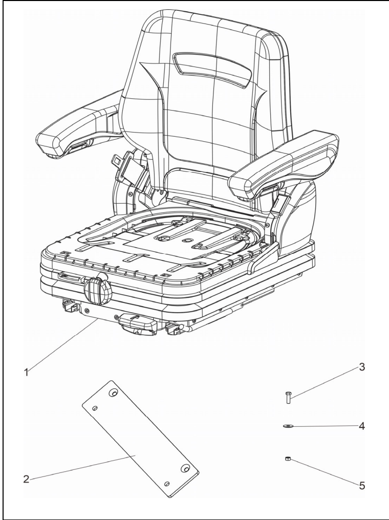
Рисунок 6-3А. Сиденье в сборе Figure 6-3A Seat assembly
