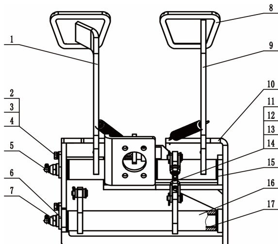
Рисунок 7-1А-1. Узел микровыключателя педали тормоза (электрогидравлическая трансмиссия) Figure 7-1A-1 Brake micro assembly 293911511002
