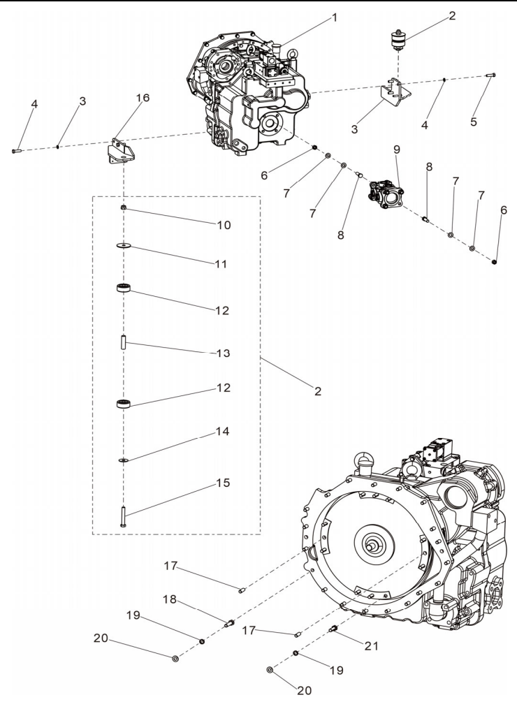
Рисунок 1-3В. Коробка передач в сборе (электрогидравлическая, двигатель S6S) Figure 1-3B Transmission assembly
