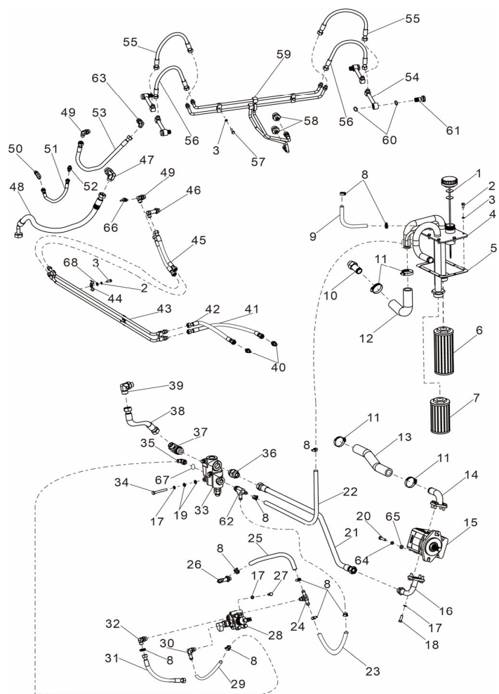
Рисунок 9-2. Гидравлическая система шасси (механическая трансмиссия) Figure 9-2 Body Hydraulic System
