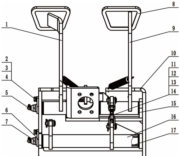
Рисунок 8-2-1. Узел микровыключателя педали тормоза (S6S) Figure 8-2-1 Brake Micro Assembly 293911511003
