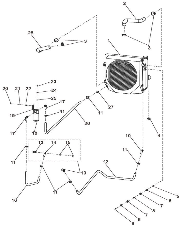
Рисунок 5-3. Радиатор в сборе (S6S) Figure 5-3 Radiator Assembly (S6S)
