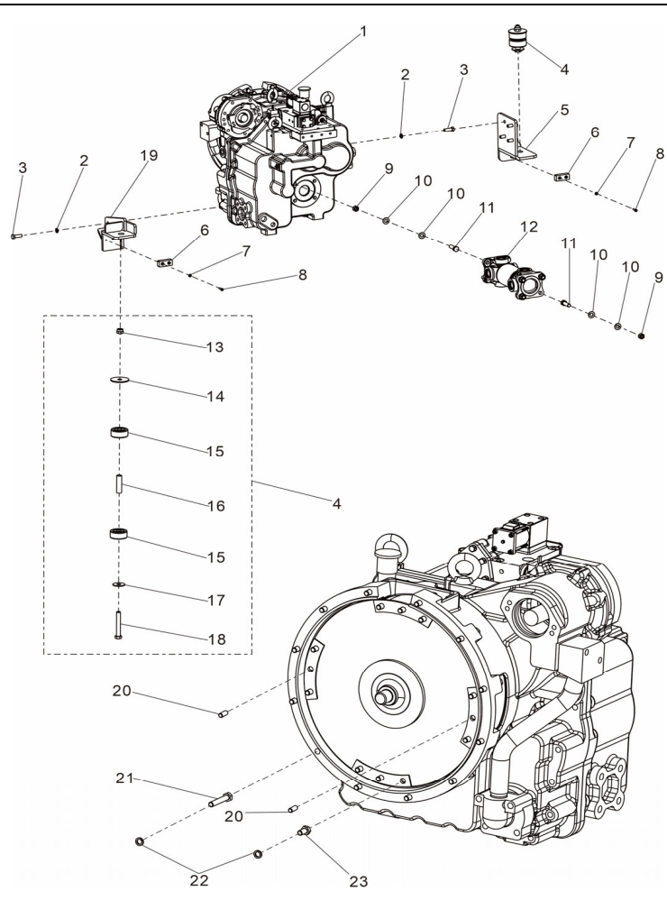
Рисунок 1-3А. Коробка передач в сборе (электрогидравлическая) Figure 1-3A Transmission assembly
