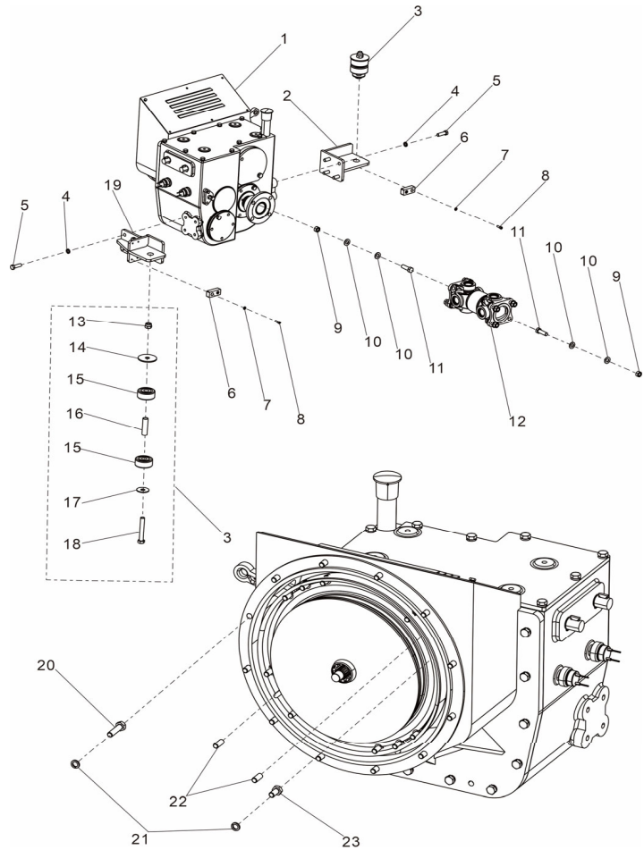
Рисунок 1-3. Коробка передач в сборе (механическая) Figure 1-3 Transmission assembly
