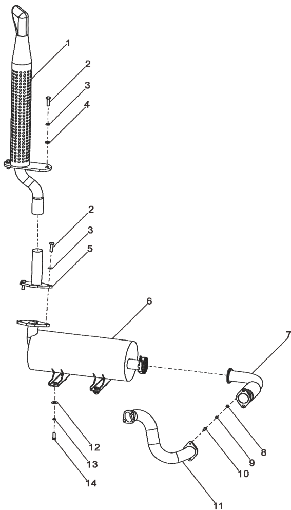
Рисунок 5-2. Глушитель в сборе (двигатель S6S, высокое расположение выхлопной трубы) Figure 5-2 Muffler Assembly (S6S high row)
