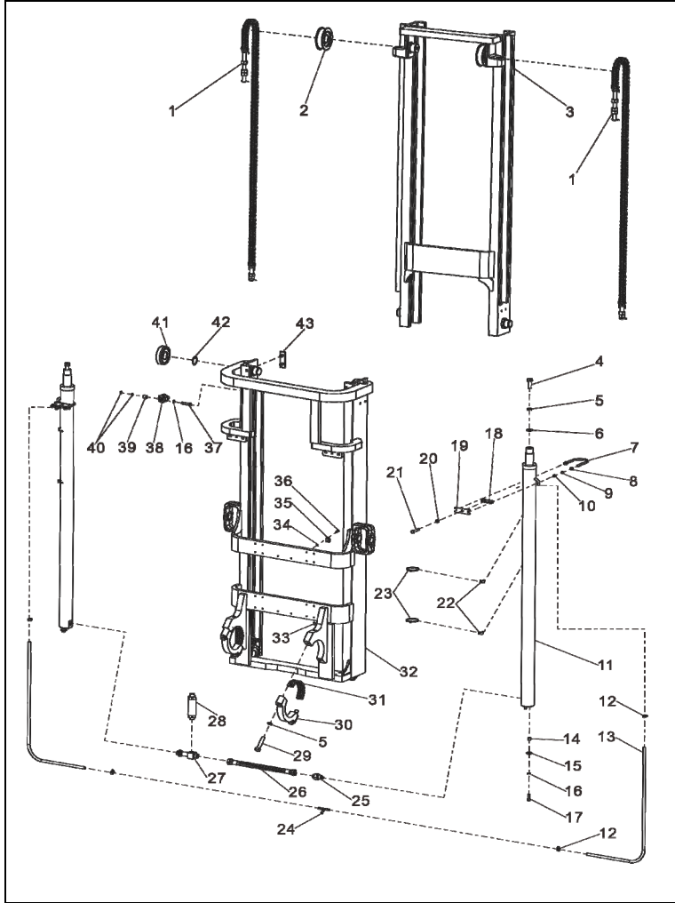
Рисунок 10-1. Двухсекционная мачта в сборе Figure 10-1 Secondary frame assembly
