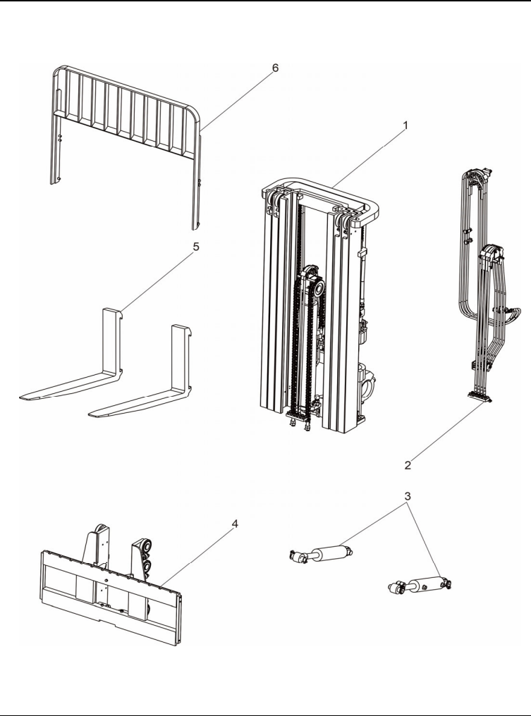
Рисунок 11. Трехсекционная мачта Figure 11 Three level gantry system
