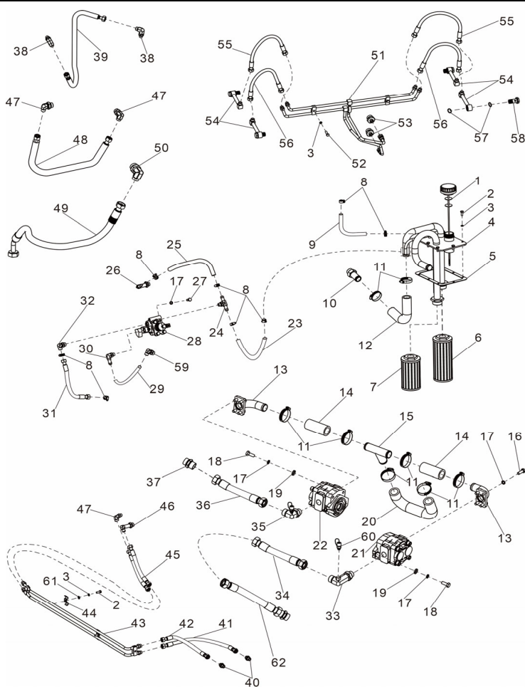
Рисунок 9-2В. Гидравлическая система шасси (двигатель S6S, электрогидравлическая трансмиссия) Figure 9-2B Body hydraulic system
