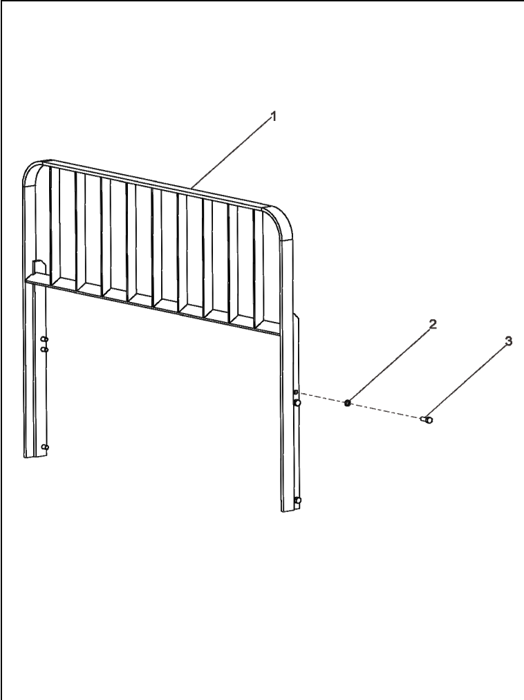
Рисунок 10-6. Защитная решетка груза в сборе Figure 10-6 Rack assy
