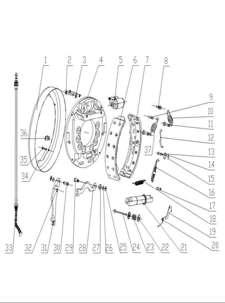
Рисунок 1-1-1-2. Тормозной механизм в сборе (левый) FH45LY-705-A1280 Figure 1-1-1-2 Brake assembly 293998510006
