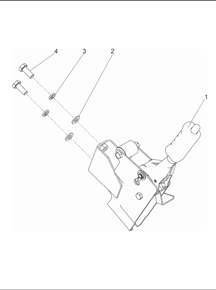
Рисунок 7-4. Стояночная тормозная система в сборе Figure 7-4 Parking brake assembly
