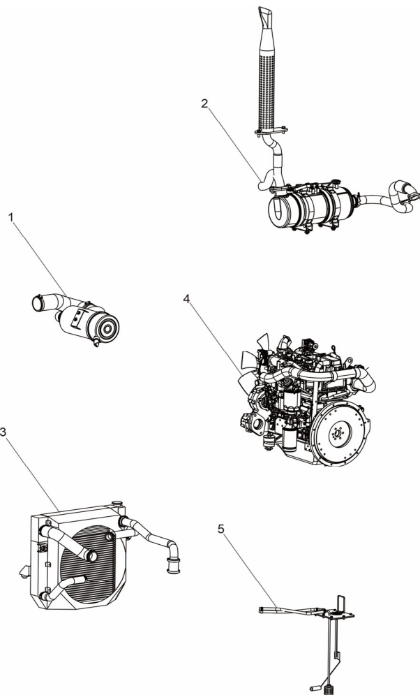
Рисунок 3. Силовая установка (двигатель V35-88C41, механическая трансмиссия) Figure 3 Power system
