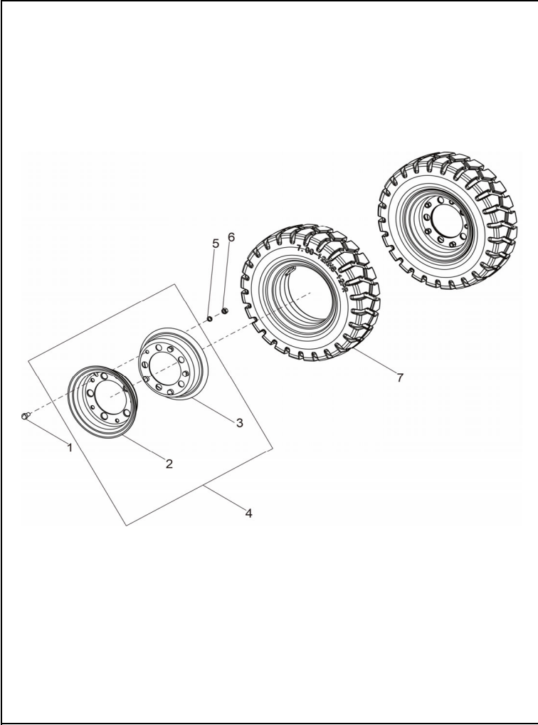
Рисунок 2-2. Управляемое колесо в сборе Figure 2-2 Steering wheel assembly
