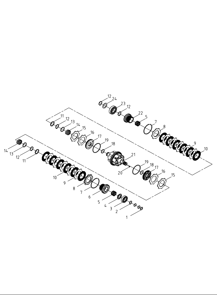
Рисунок 1-3А-1-1. Муфта сцепления первичного (входного) вала в сборе SDT45-02000 Figure 1-3A-1-1 Input shaft clutch assembly 293998510001
