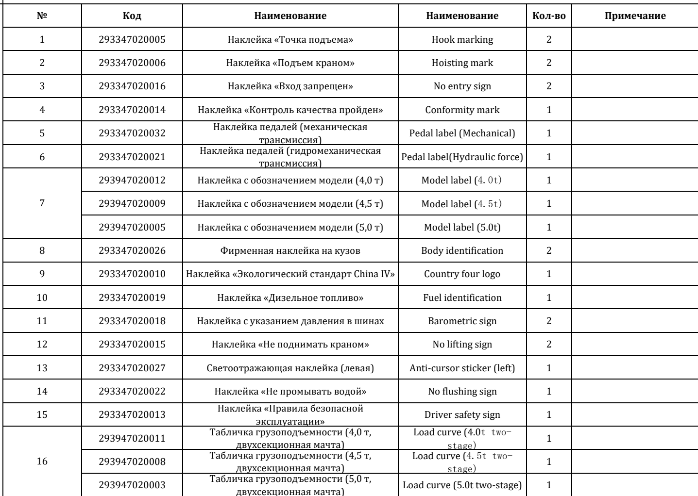
A#CPC40-A02,B#CPC45-A02,C#CPC50-A02,D#CPCD40-A02,E#CPCD45-A02,F#CPCD50-A02,G#CPCD40-AS3,H#CPCD45-AS3,I#CPCD50-AS3
