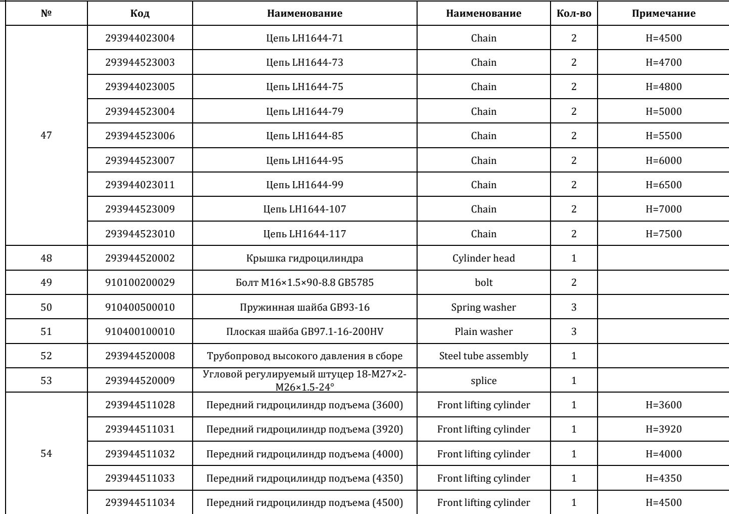
A#CPC40-AQ2,B#CPC45-AQ2,C#CPC50-AQ2,D#CPCD40-AQ2,E#CPCD45-AQ2,F#CPCD50-AQ2,G#CPCD40-AS3,H#CPCD45-AS3,I#CPCD50-AS3
